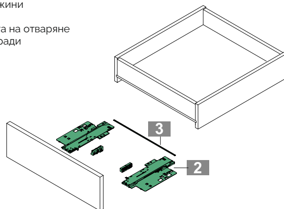
Позиция на синхронизиращата шина
