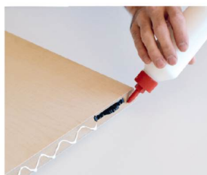
3. Нанасяне на лепило
