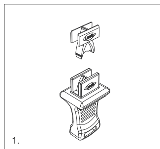
1. Поставете помощния клипс в инструмента
